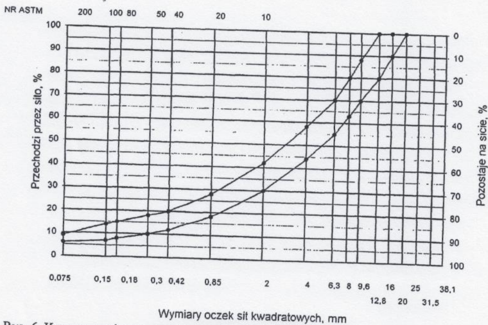
Wymiary oczek sit kwadratowych, mm Rys. 5. Krzywe graniczne uziarnienia mieszanki mineralnej BA od 0 do 20 mm (mieszanka o nieciągłym uziarnieniu) do warstwy ścieralnej nawierzchni drogi o obciążeniu ruchem od KR3 do KR6
